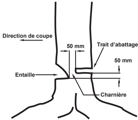
Figure BB.102 - Description de l'abattage: exécution de l'entaille
